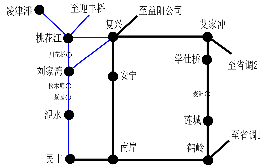
省网A2平面光纤通信网络现状图
