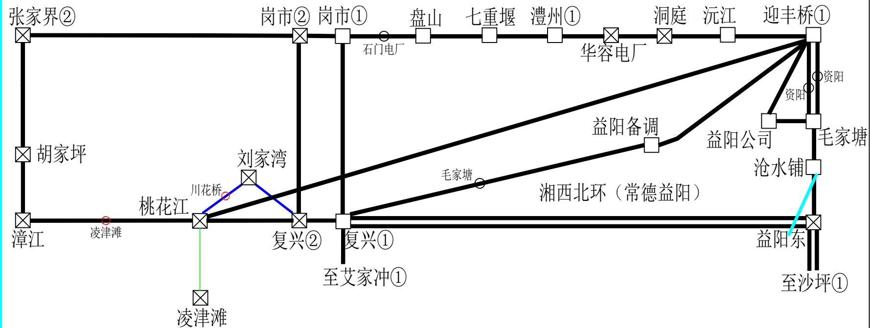
省网A1平面光纤通信网络组织图
